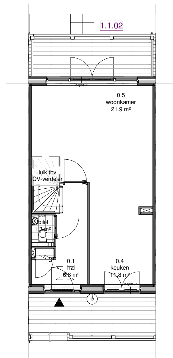
Begane grond - Veranda 1800mm optie nr.: 1.1.02 (alle types)
