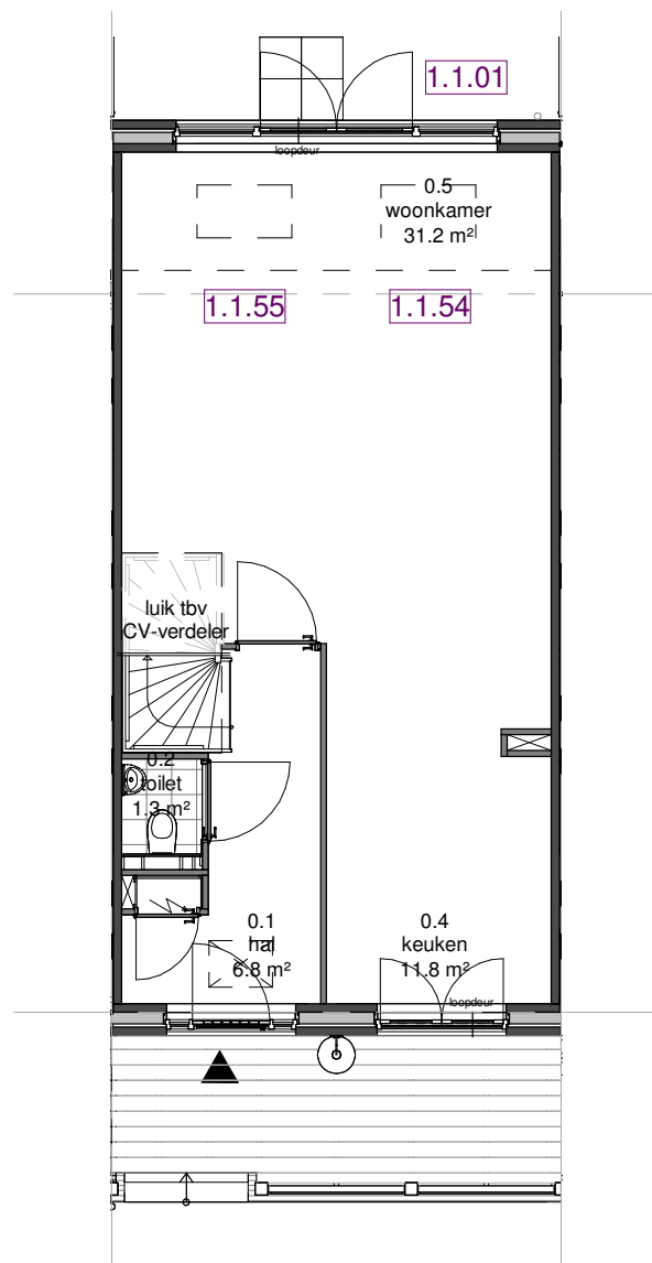
Begane grond - Aanbouw 1800mm optie nr.: 1.1.01 (alle types)
